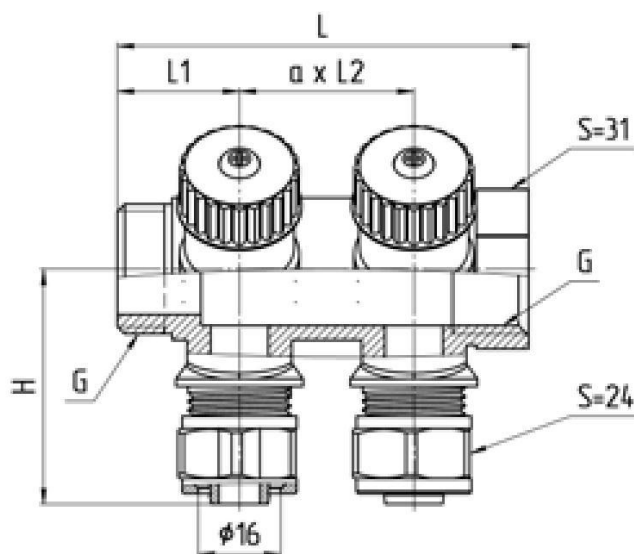
Рисунок 2 –Габаритные размеры коллектора
