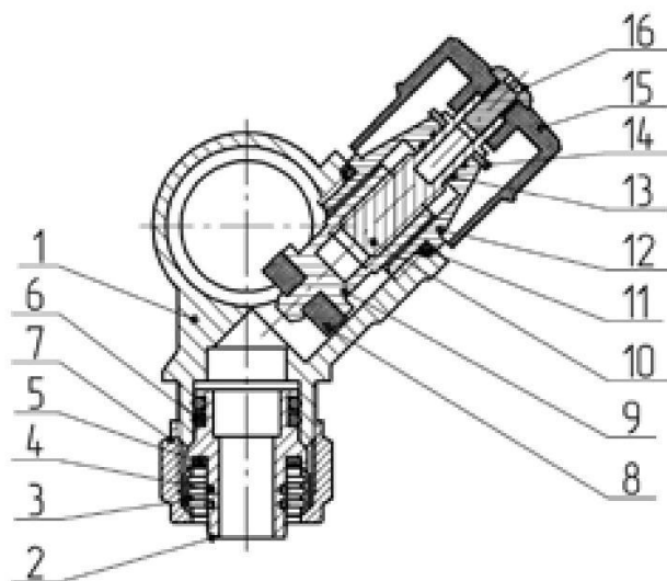
Рисунок 1 – Конструкция коллектора с регулирующими клапанами
